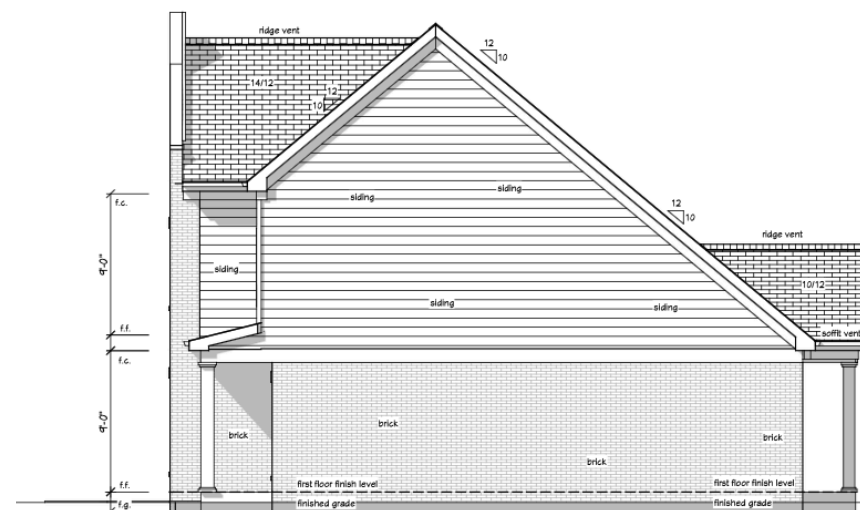
right elevation scale: 1/4" = 1'-0"
