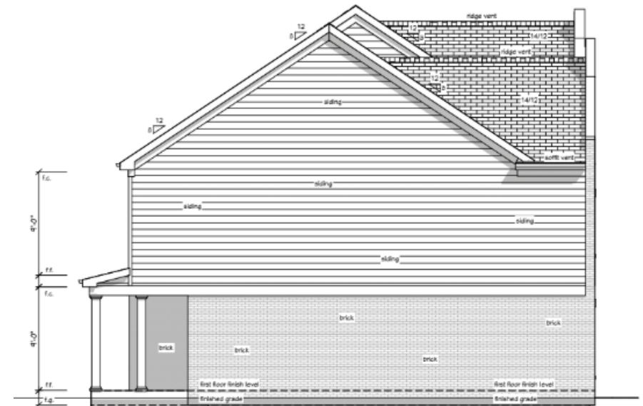
left elevation scale: 1/4" = 1'-0"
