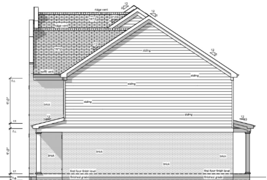
right elevation scale: 1/4" = 1'-0"
